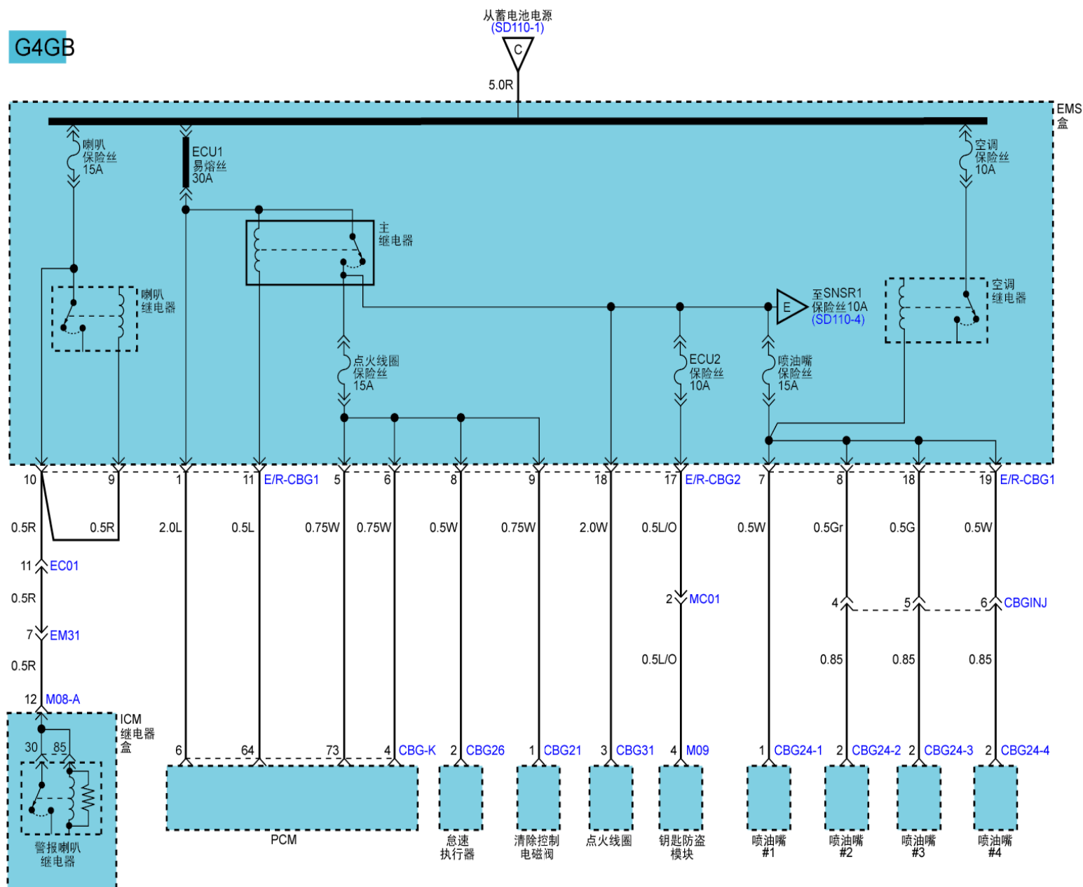
电源分布(3)
