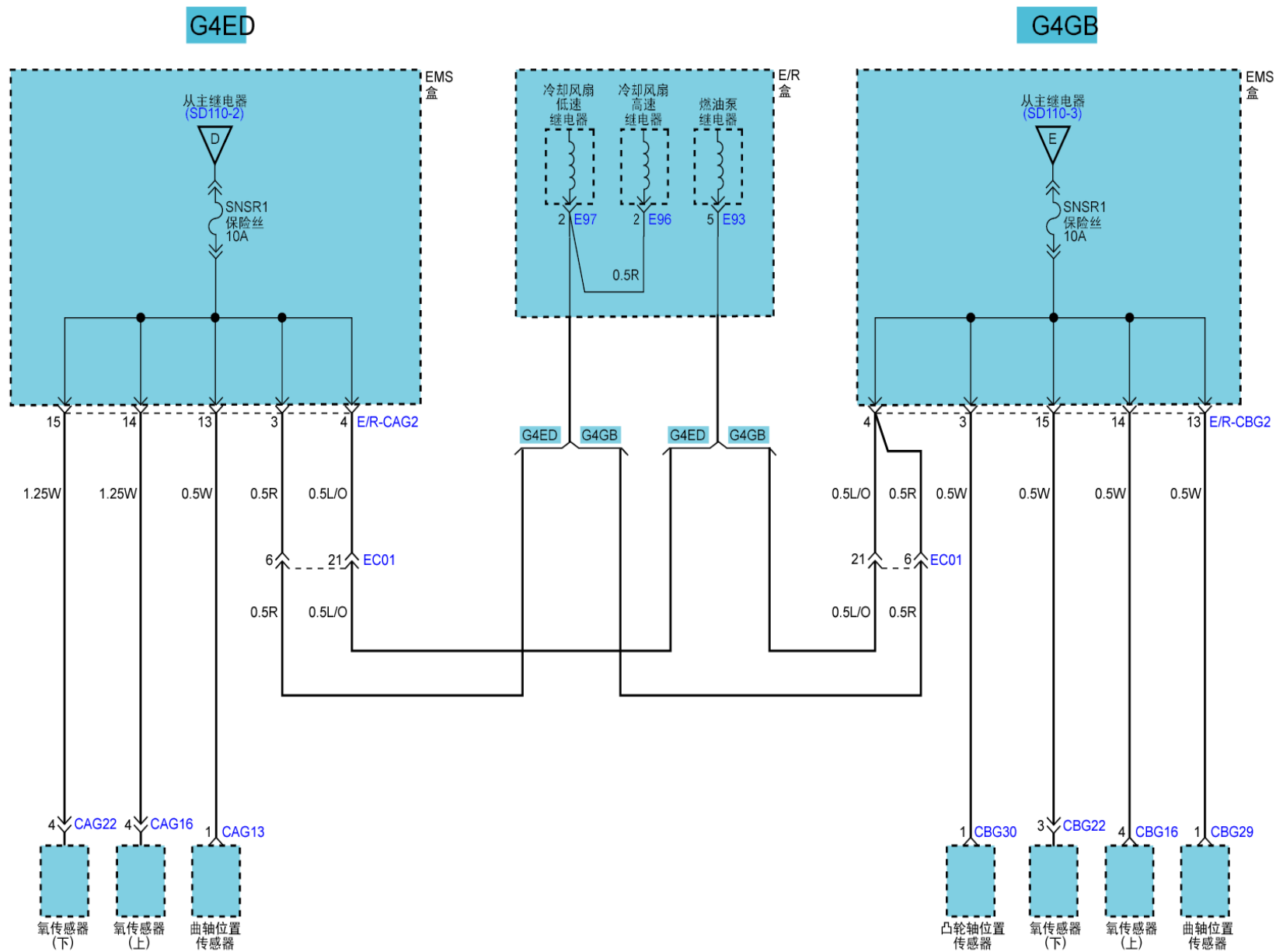
电源分布(4)
