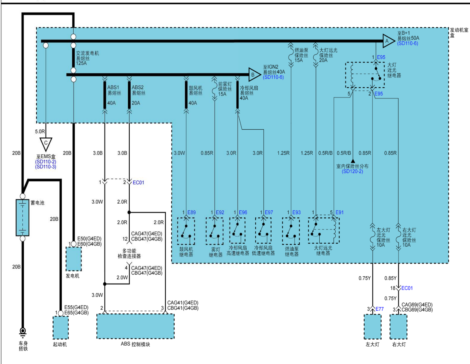
电源分布(1)
