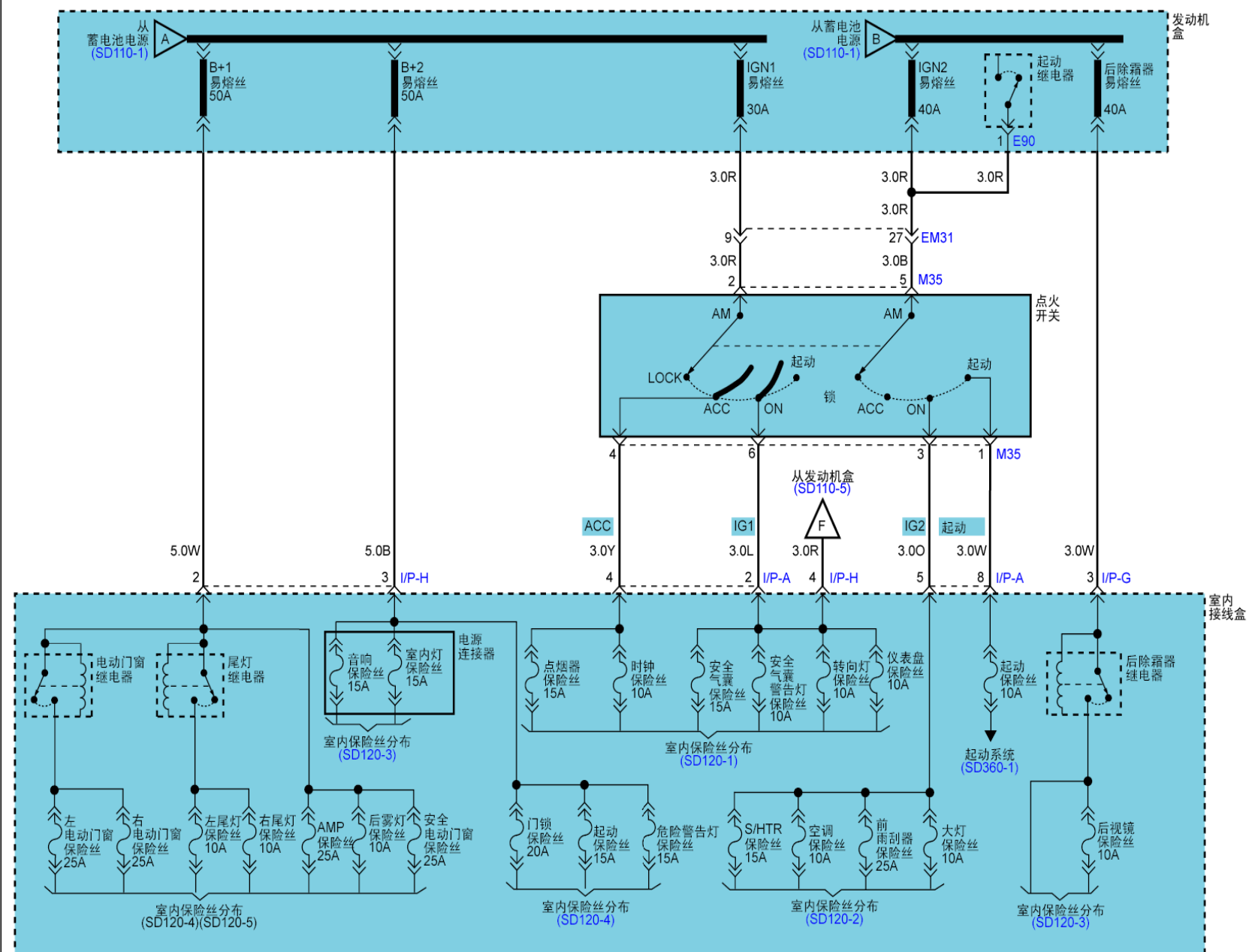
电源分布(6)
