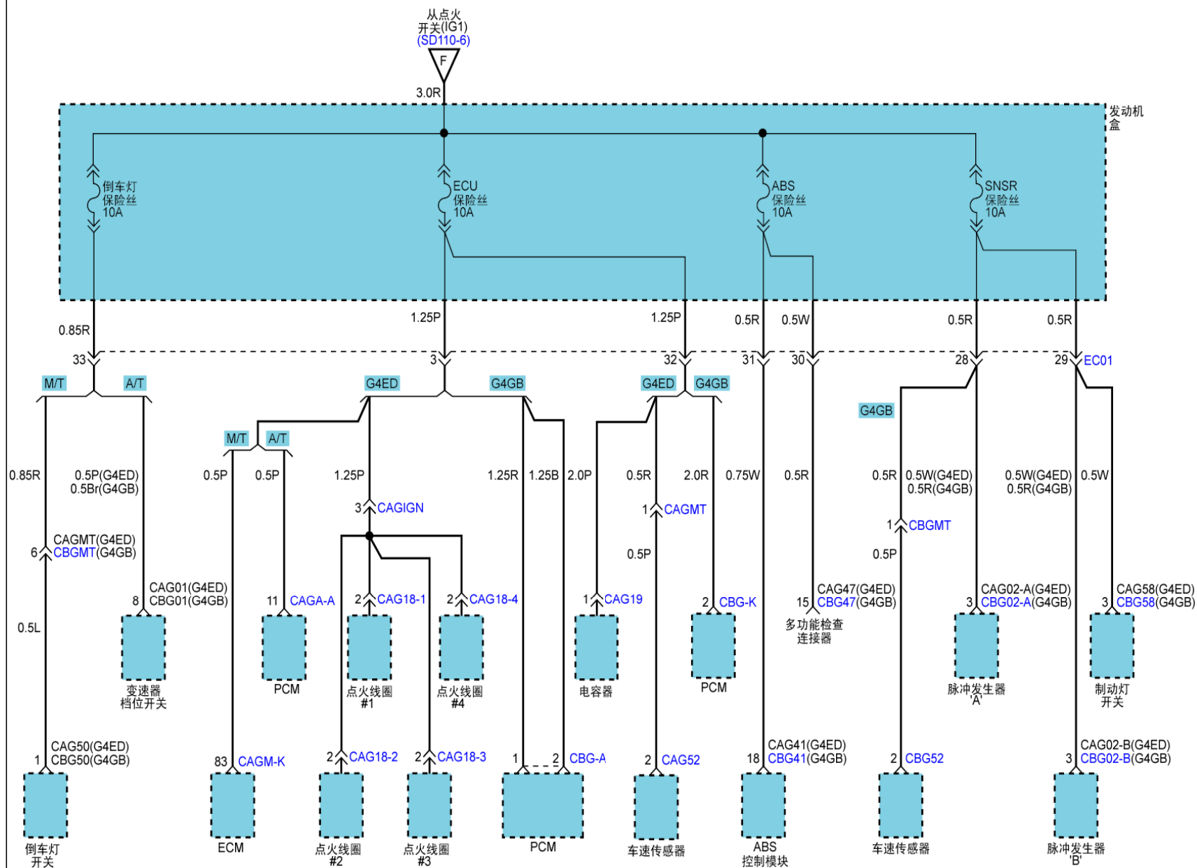
电源分布(5)
